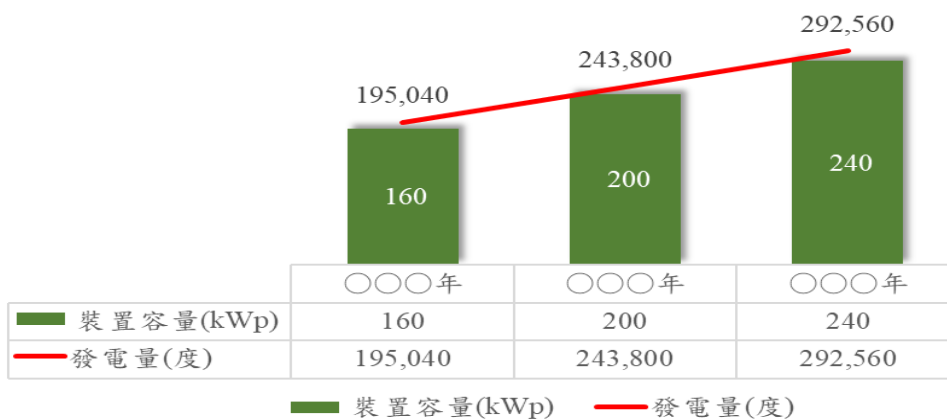
近 3 年太陽能系統發電量比較
